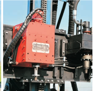
Particolare gruppo testata modello JOY 2 / JOY 2 Sight head set
