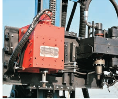
Groupe spécial tête modèle JOY 2 Teilansicht Kopfgruppe Modell JOY 2
