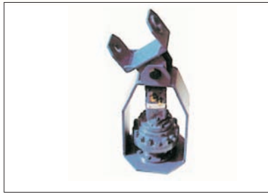
Tête mod. T3 dotée de châssis et de double articulation. Bohrkopf Mod. T3 komplett mit Rahmen und Doppelgelenk.
